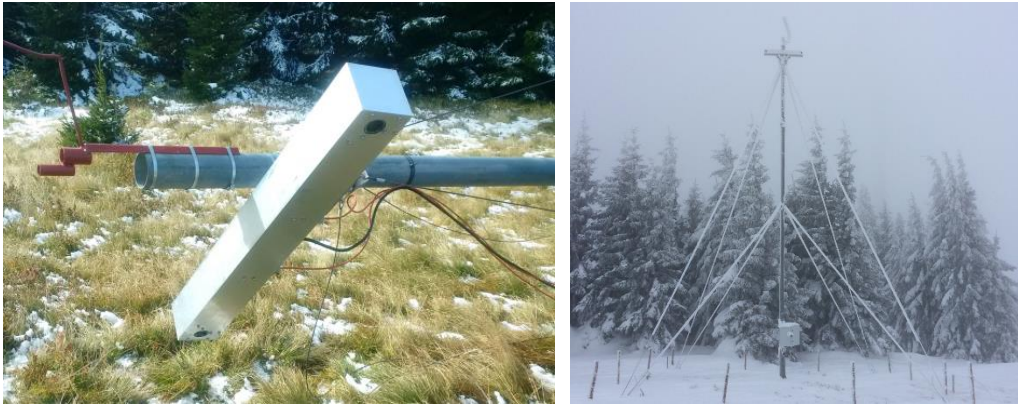
Abbildung 3: Kamerabasiertes 3D-Messsystem: Montage des Messsystems auf umgelegtem Messturm (links), Messturm mit Messsystem bei winterlichen Bedingungen (rechts)
